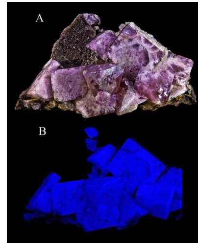
Fluorit-Kristalle im UV-Licht
