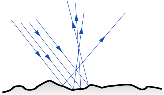
diffuse Reflexion
