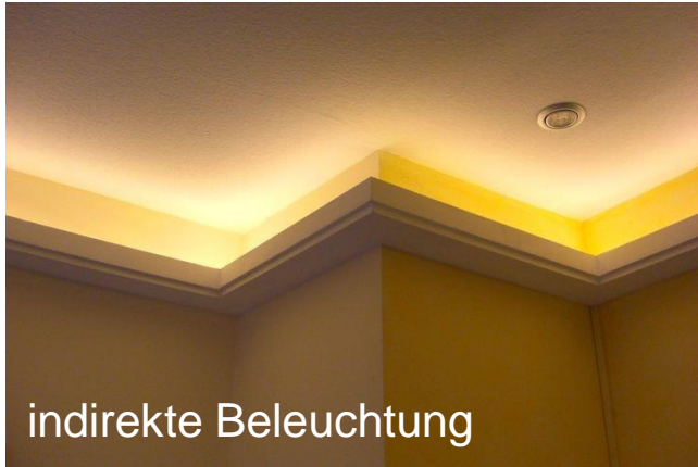
diffuse Reflexion
